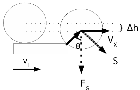
図1: 机のかどの球の状態
