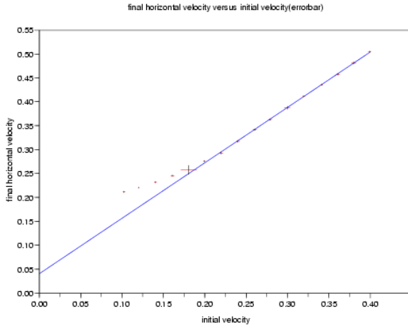
図 2: 球の初速度と落下中の球の速度の水平成分
