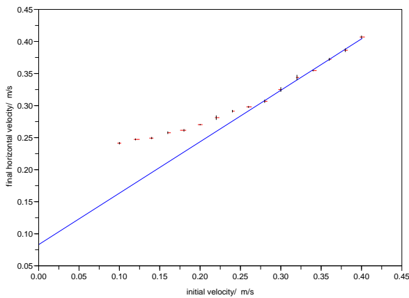
図 3: 円柱の初速度と落下中の円柱の速度の水平成分
